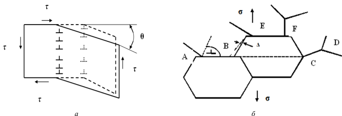
Рисунок 1 – Схема движения малоугловой границы зерна с одной степенью свободы под действием напряжения \tau (а) и совместной пластической деформации зернограничного проскальзывания и внутризеренного скольжения (б)
