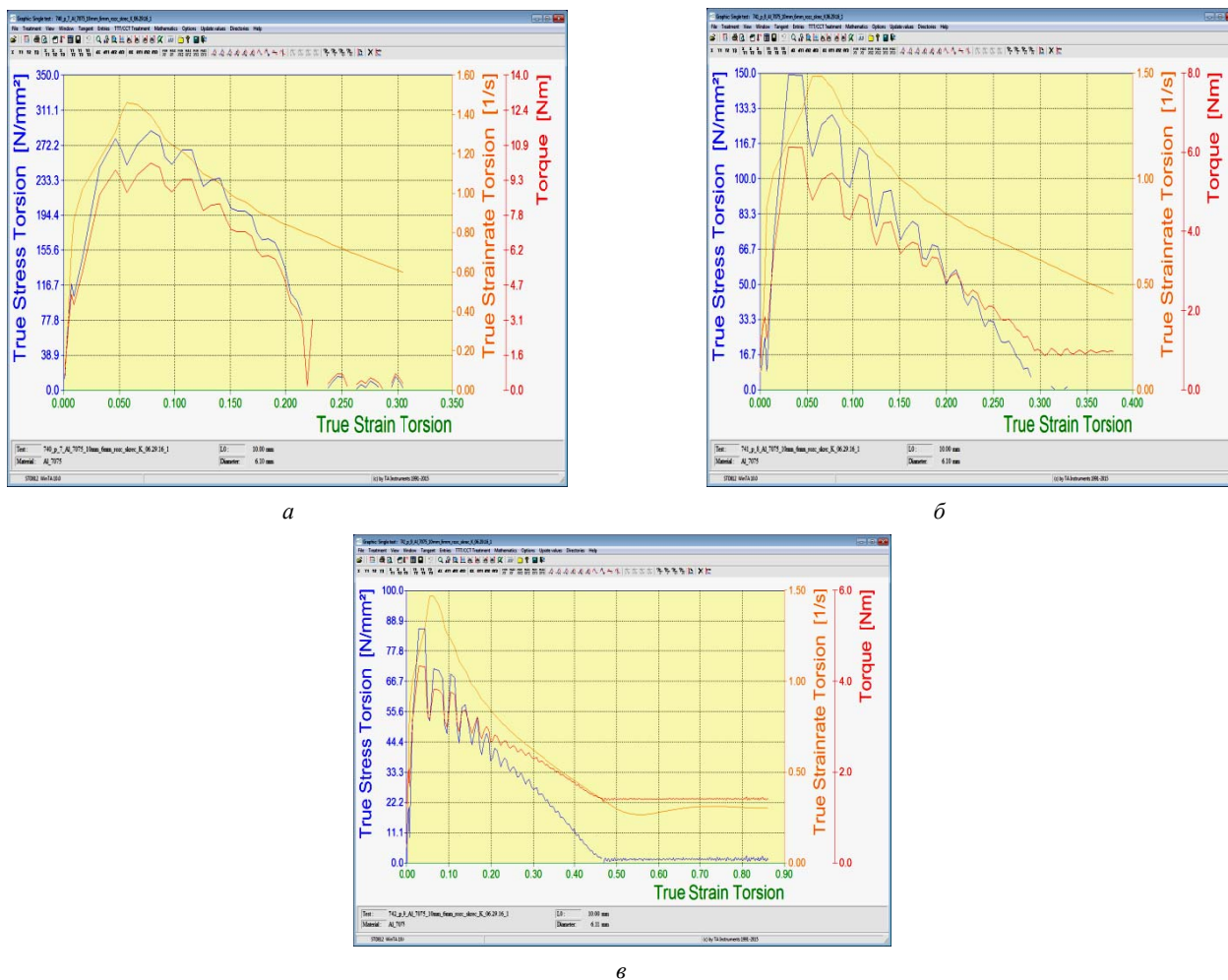
Рисунок 5 – Влияние растяжений при скручивающем растяжении на изменение сопротивления деформации алюминиевого сплава 7075: a – 200 °С; б – 300 °С; в – 400 °С
