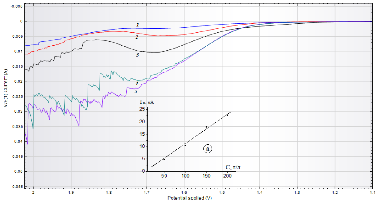
3-сурет – Родий электродының тұз қышқылы ерітінділеріндегі анодты потенциодинамикалық поляризациялық қисықтары (а – анодтық максимум ток мәндерінің тұз қышқылы концентрациясына тәуелділігі): v = 50 \text{ мВ/с} ; t = 25 \text{ }^\circ\text{C} ; \text{HCl} , г/л: 1 – 25; 2 – 50; 3 – 100; 4 – 150; 5 – 200
