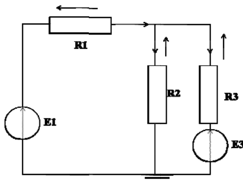
Рисунок 2 – Расчетная схема цепи постоянного тока.
