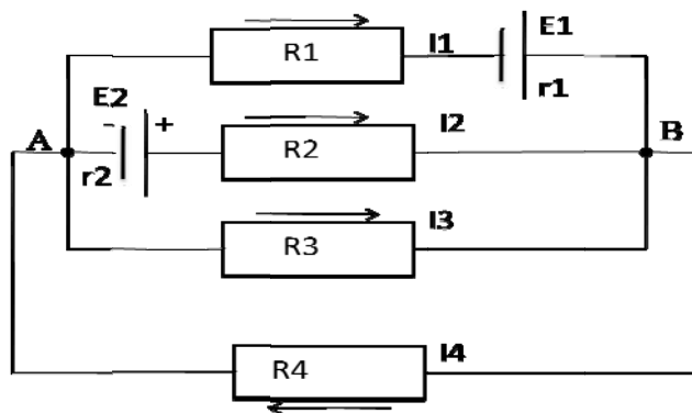
Рисунок 1 – Разветвленная электрическая цепь с источниками
