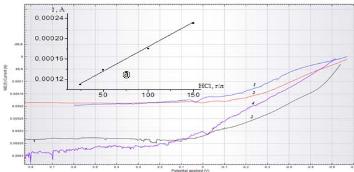
1-сурет – Таллий электродында түсірілген анодты потенциал-динамикалық поляризациялық қисығы (а – таллий электродының потенциалы «минус» 0,3 В болған кезде оның еру тоғы мәндерінің тұз қышқылы концентрациясына тәуелділігі)
